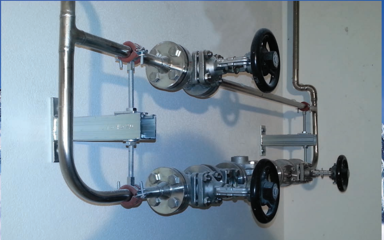
Konsolenhalterung für Absperrhähne Konsolle 45/45/2,0 längs
